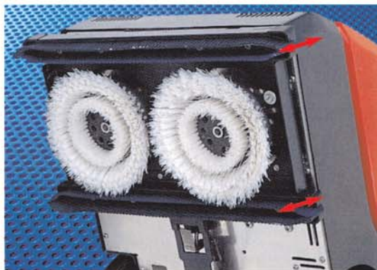
RA 300 E: Abhebbare Sauglippen
